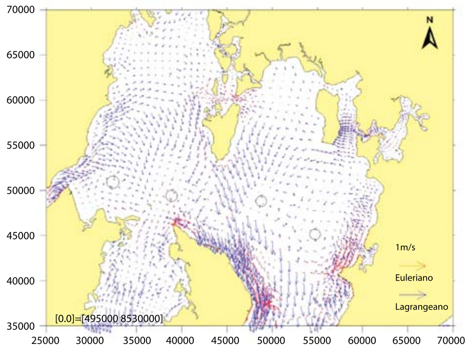
Figura 17. Padrão da circulação residual lagrangeana (em azul) e euleriana (em vermelho) na área central da BTS, ao final de dois ciclos de maré, sem considerar o cisalhamento eólico. O sentido de rotação dos vórtices residuais é também indicado (modificado de Xavier, 2002).
