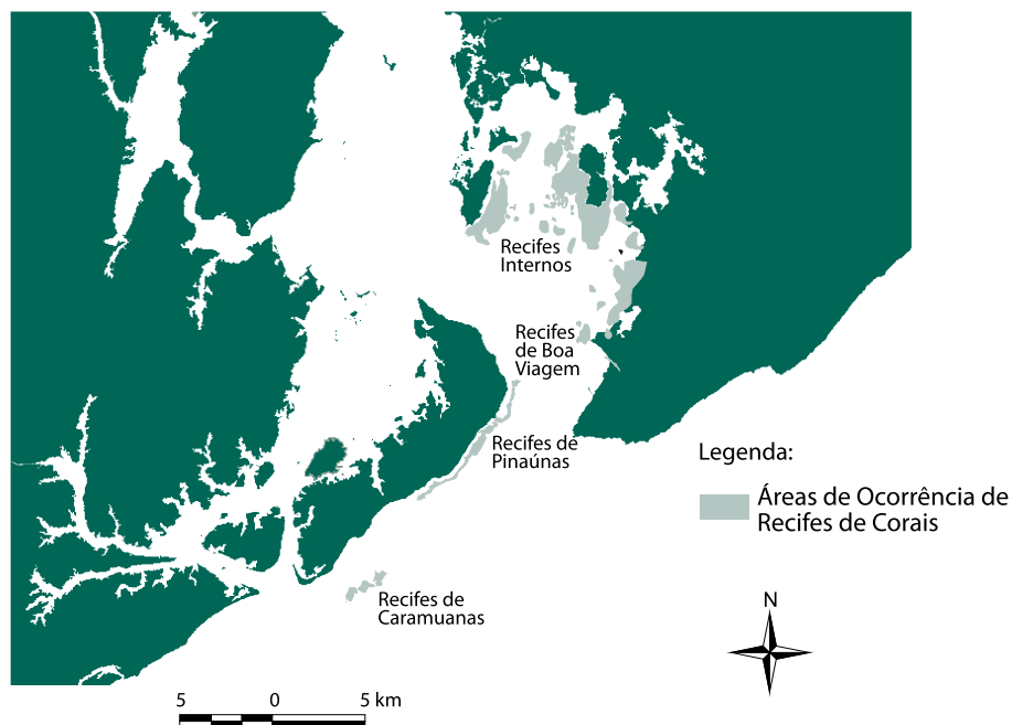
Figura 8. Localização dos recifes de corais da Baía de Todos os Santos (adaptado de Cruz, 2008).
