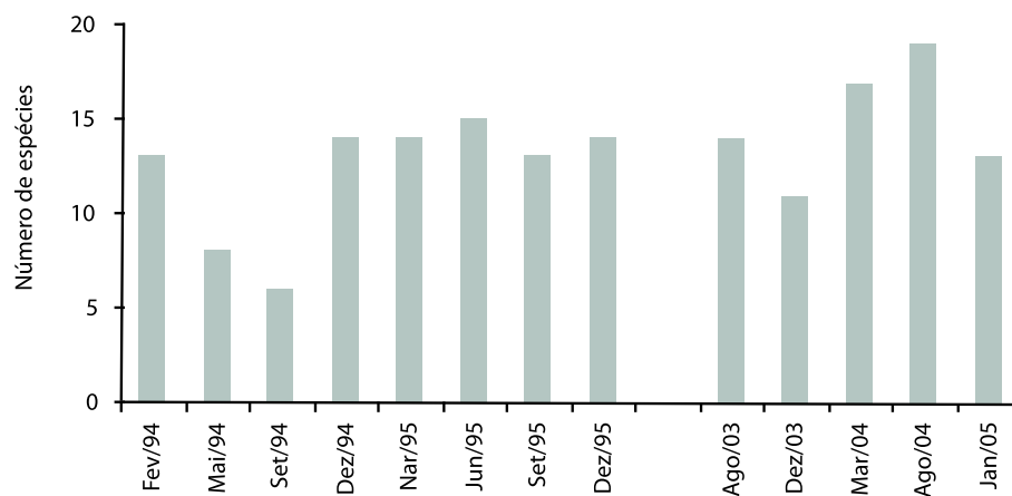
Figura 14. Valores do número de espécies da ictiofauna capturada na região adjacente a Mataripe. Os dados de fevereiro de 1994 a dezembro de 1995 referem-se às coletas do projeto ECONORTE, e os de agosto de 2003 a janeiro de 2005 ao projeto PROMARLAM.
