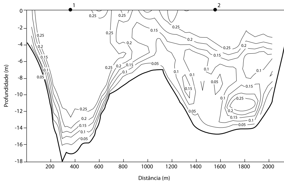
Figura 26. Campo de velocidade ( m s^{-1} ) no canal de São Roque, próximo à ilha do Francês – máximo de vazante na maré de quadratura (31/01/2004) (Genz, 2006).
