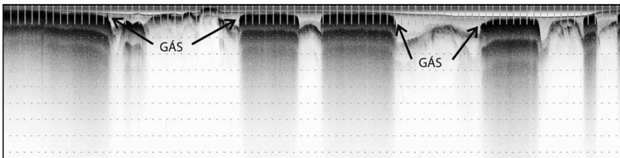
Figura 17. Exemplo de linha sísmica de alta resolução com presença de gás no sedimento (indicado pelas setas).
