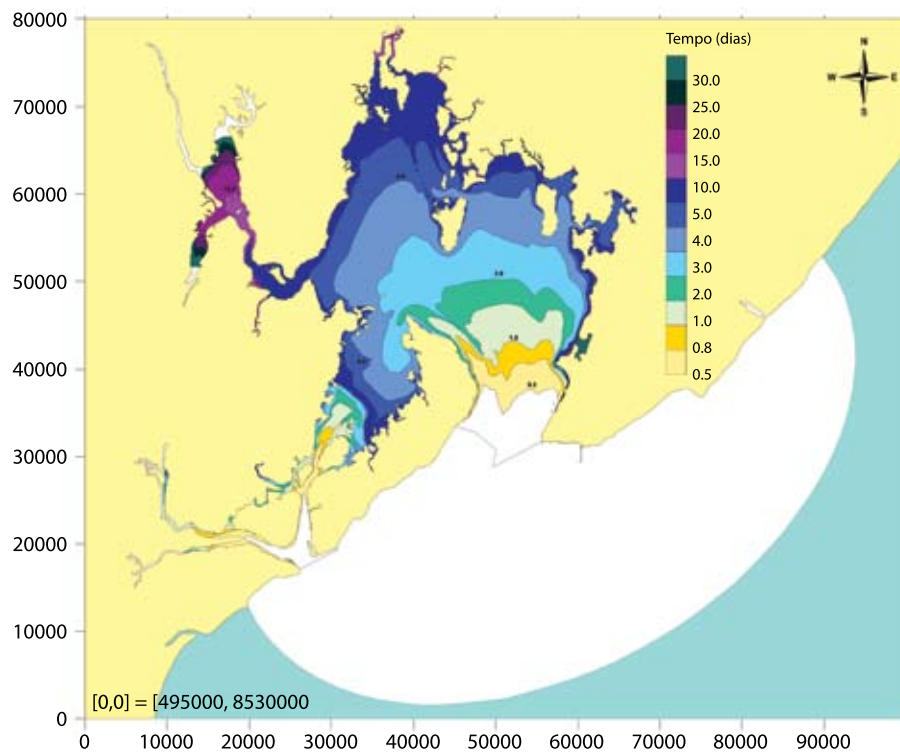
Figura 18. Zoneamento do tempo de residência na BTS, obtido através de simulação numérica do fluxo em condição de verão (maré e vento), de acordo com Xavier (2002).
