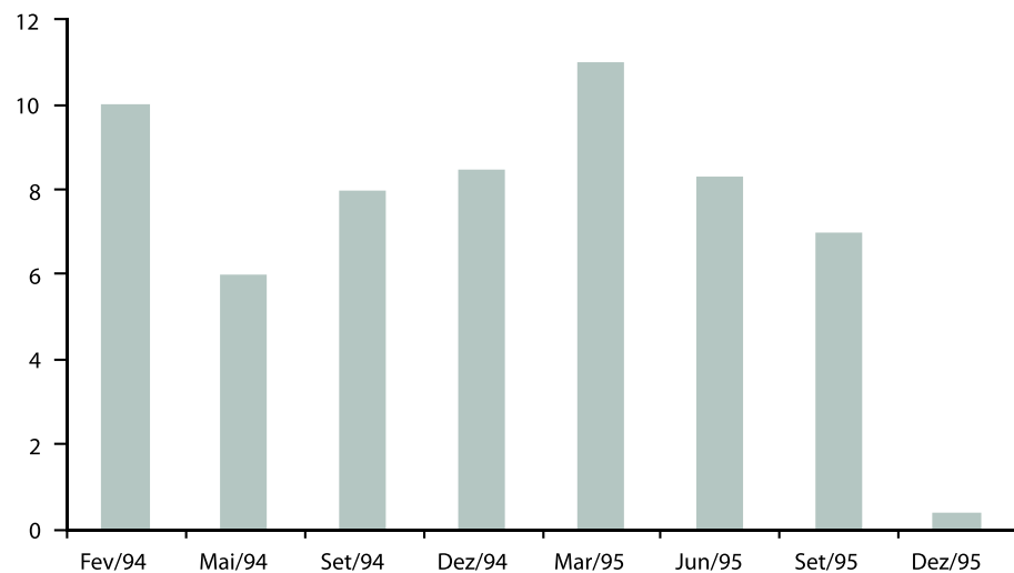
Figura 4. Variação temporal dos valores médios de silicato ( \text{mg L}^{-1} ) na BTS, durante 1994-1995 (projeto ECONORTE).
