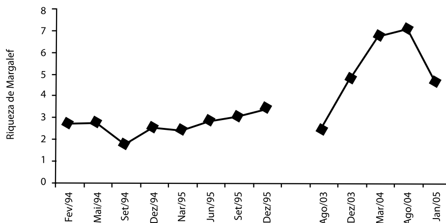
Figura 15. Valores estimados do índice de riqueza de Margalef para a ictiofauna capturada na região adjacente a Mataripe. Dados de fevereiro de 1994 a dezembro de 1995 referem-se às coletas do projeto ECONORTE e os de agosto de 2003 a janeiro de 2005 ao projeto PROMARLAM.
